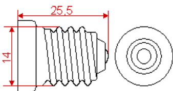
E14 Sockel-Layout E14 base layout
